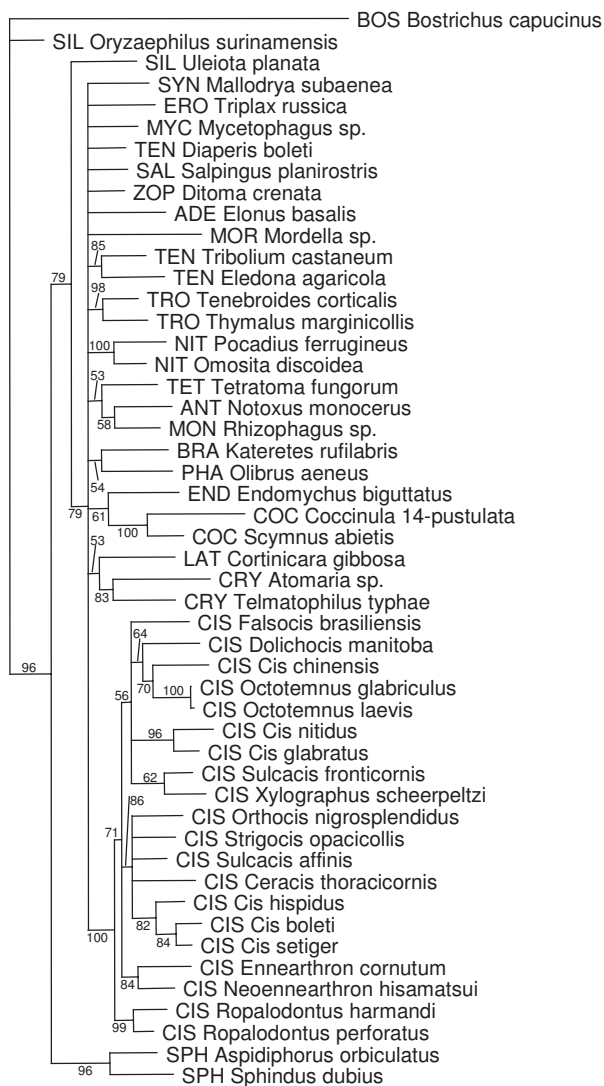
— 0.1 6 E-sample-MB[COI,18S](50%mr)
